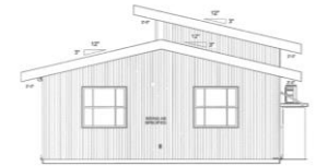
Right Elevation
