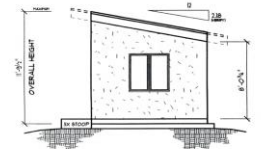
Right Elevation
